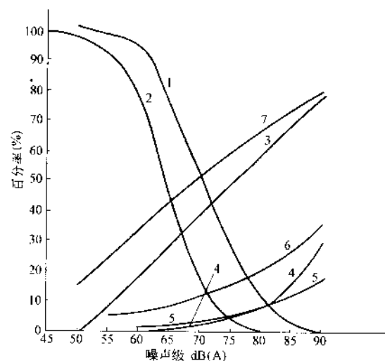
图1 洁净厂房噪声分布与评价图
