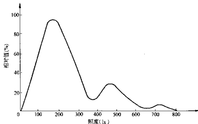
图 3 洁净车间工作面上的最低照度
