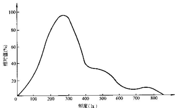
图4 洁净车间工作面上的平均照度
