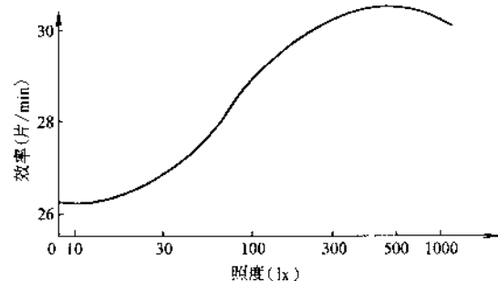
图5 不同荧光灯照度下的挑片效率
